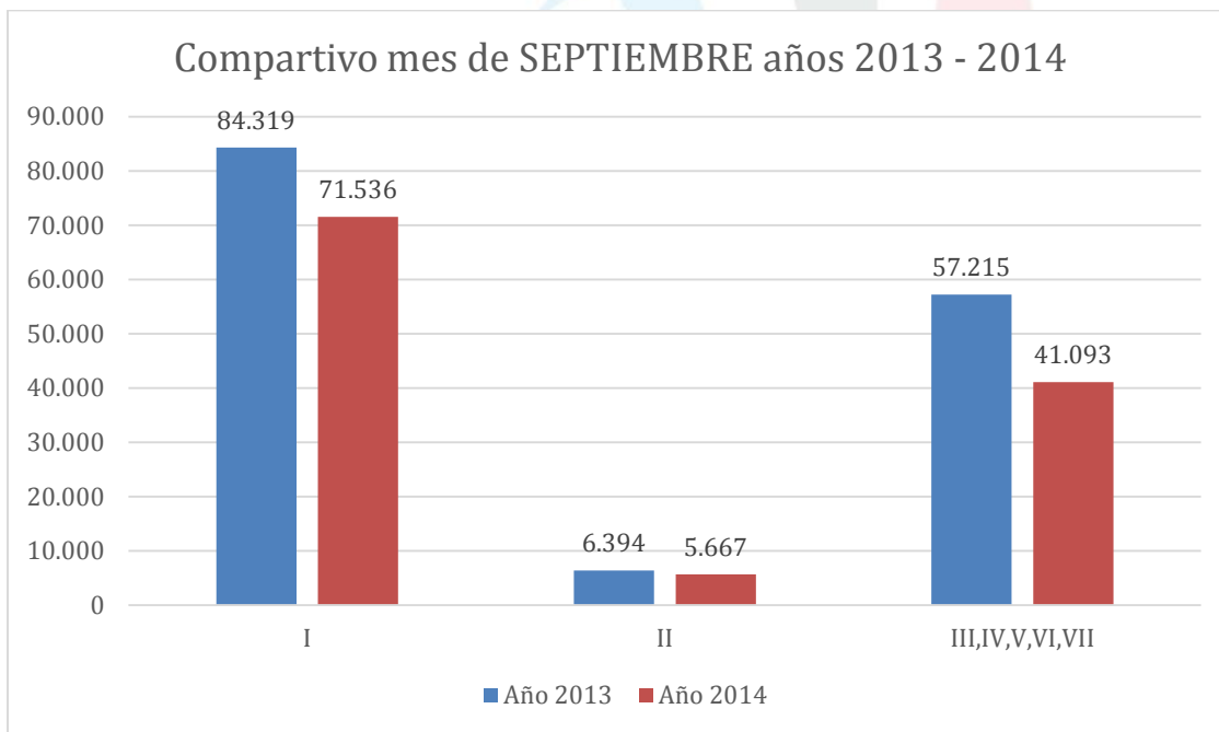
Grafica 11. Flujo vehicular peaje libertad mes de septiembre 2013/2014
